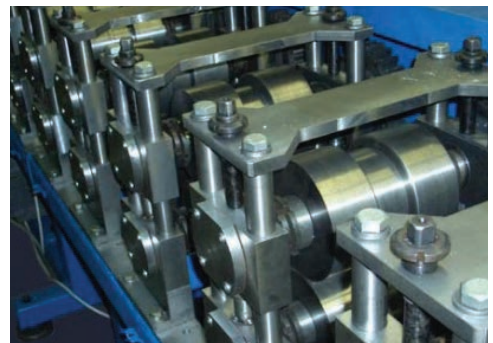
Мал. 15.14. Фальцпрокатний верстат
