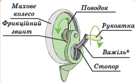
Мал. 152. Вудова ручного привода
