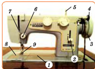
Мал. 158. Будова швейної машини
